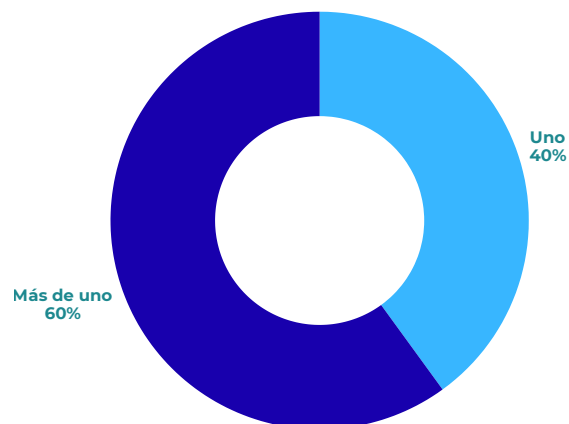
Número de agresores por incidencia
