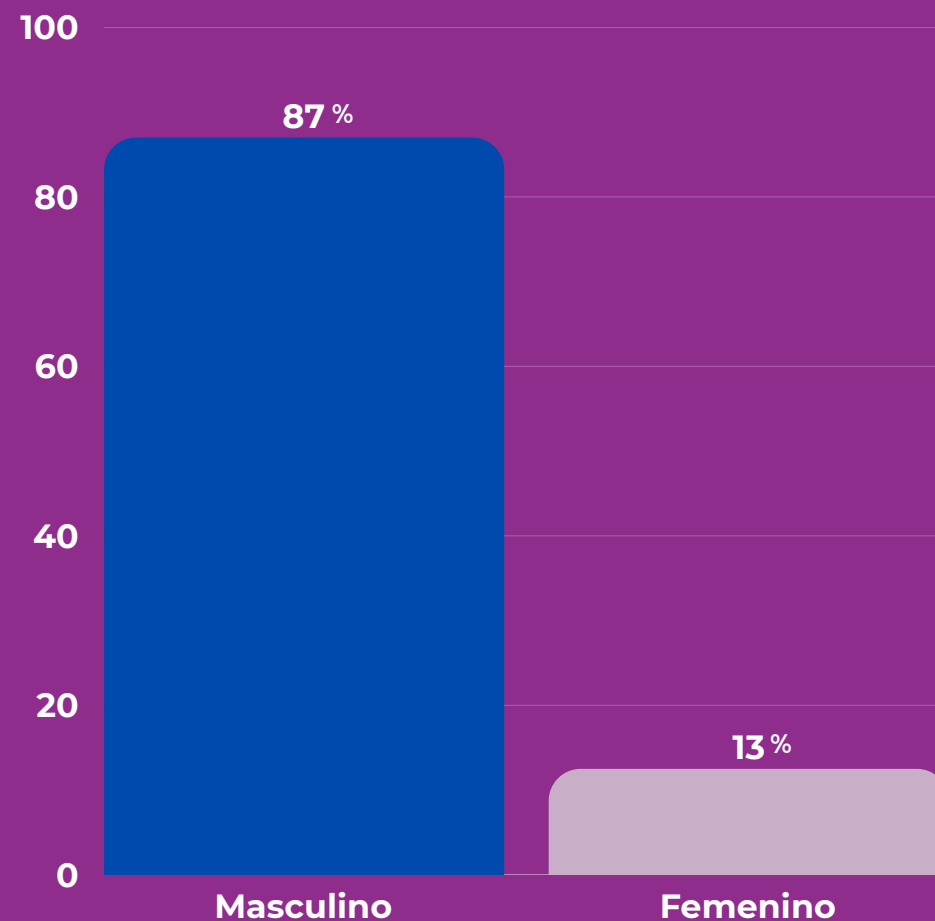
Agresores por género
