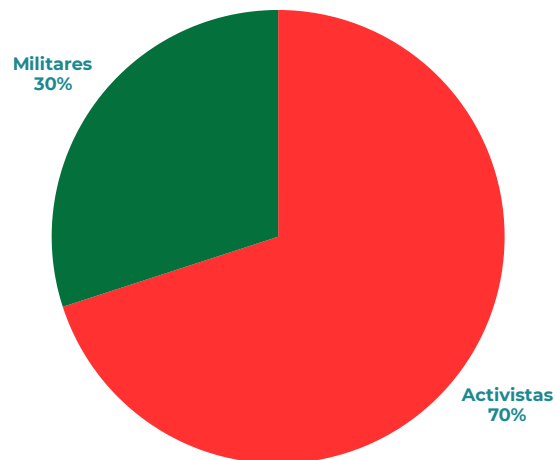
Registro de agresores por categoría
